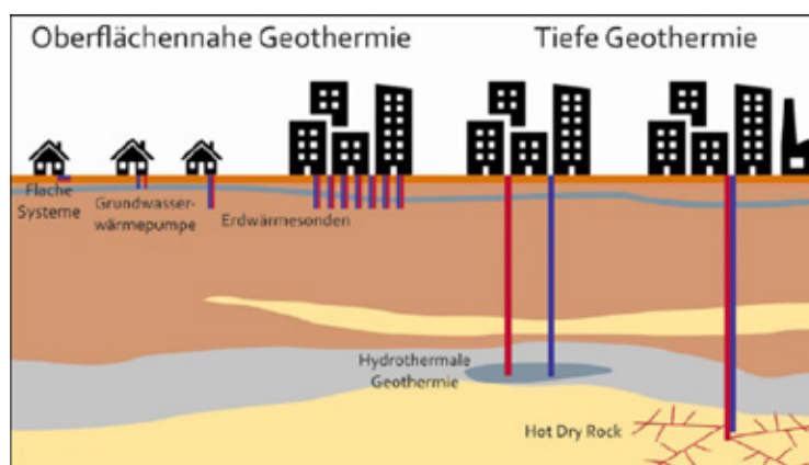
Verschiedene Varianten der Geothermie
